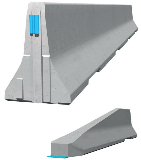
Ändelement RB80H_4T (lutning 1:5)
